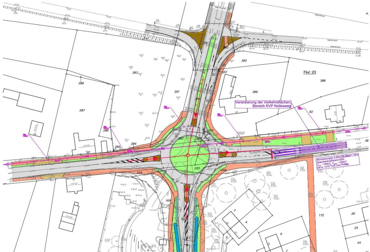
Lageplanausschnitt Bereich KVP Roermonder Straße / Nollesweg (Schemadarstellung)
