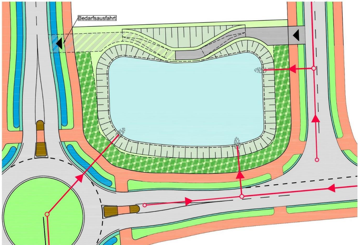
Lageplanausschnitt Bereich zentrale Mulde RQ 4 (Schemadarstellung)
