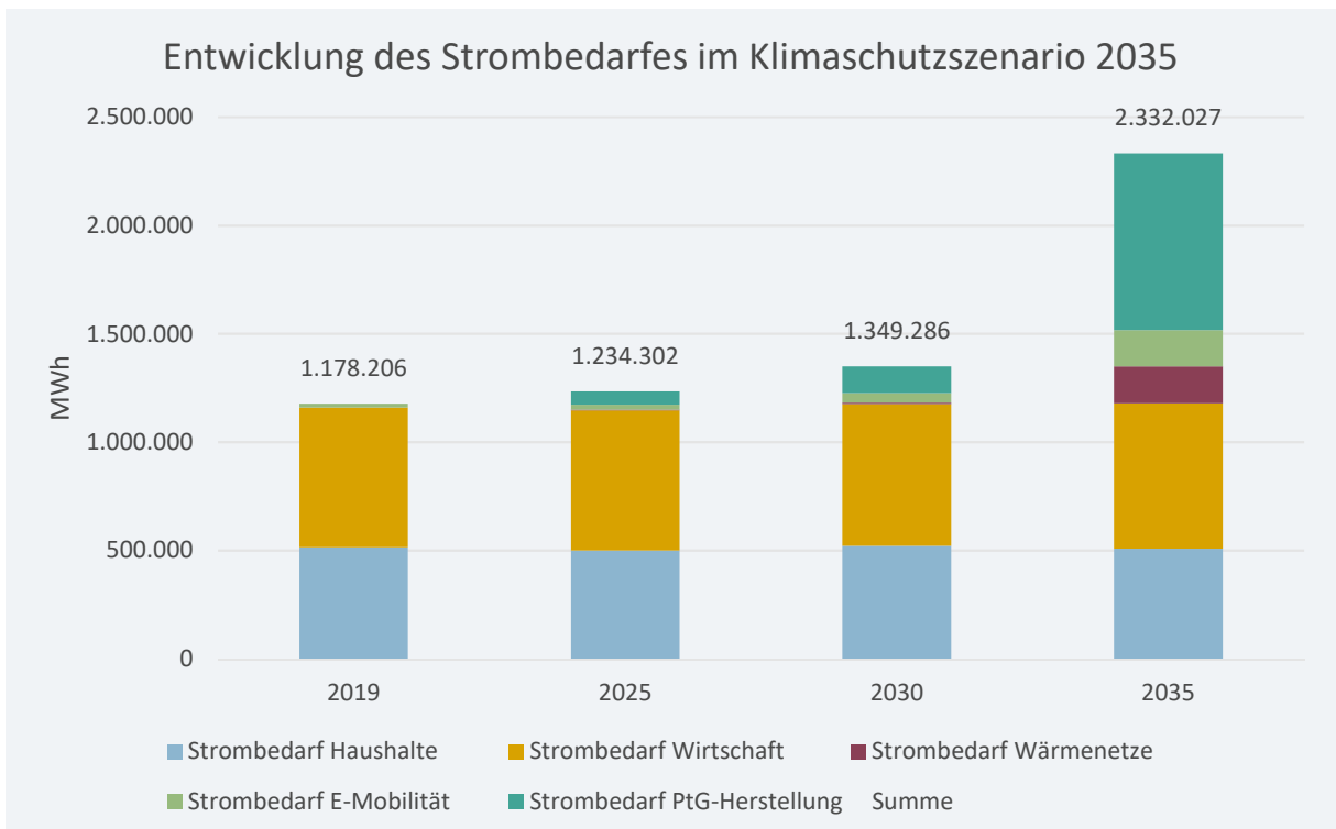
Abbildung 5-9: Entwicklung des Strombedarfes im Klimaschutzscenario 2035 inklusive E-Mobilität und Umweltwärme im Kreis Viersen (Quelle: Eigene Darstellung)
