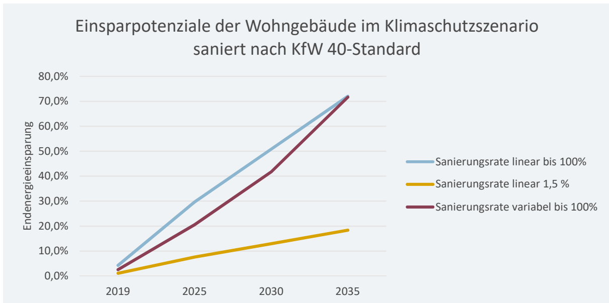
Abbildung 4-56: Einsparpotenziale der Wohngebäude „Klimaschutzscenario 2035“ (KfW 40-Standard)“ saniert bis 2035 in der Gemeinde Niederkrüchten (Quelle: Eigene Darstellung)
