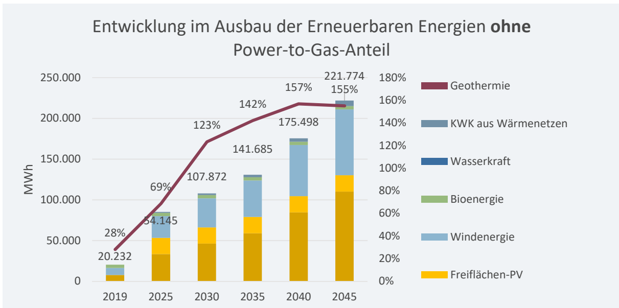
Abbildung 5-24: Entwicklung der erneuerbaren Energien im Klimaschutzscenario 2045 ohne PtG-Anteil in der Burggemeinde Brügglen (Quelle: Eigene Darstellung)
