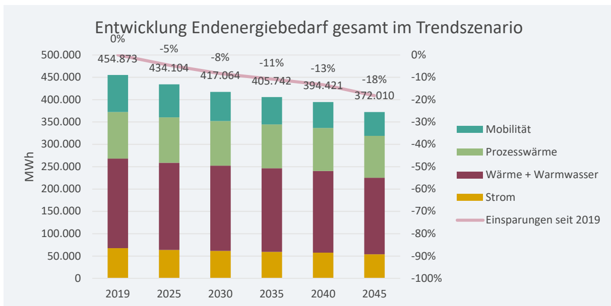
Abbildung 6-7: Entwicklung des Endenergiebedarfes nach Verwendung im Trendszenario in der Gemeinde Brügggen (Quelle: Eigene Darstellung)
