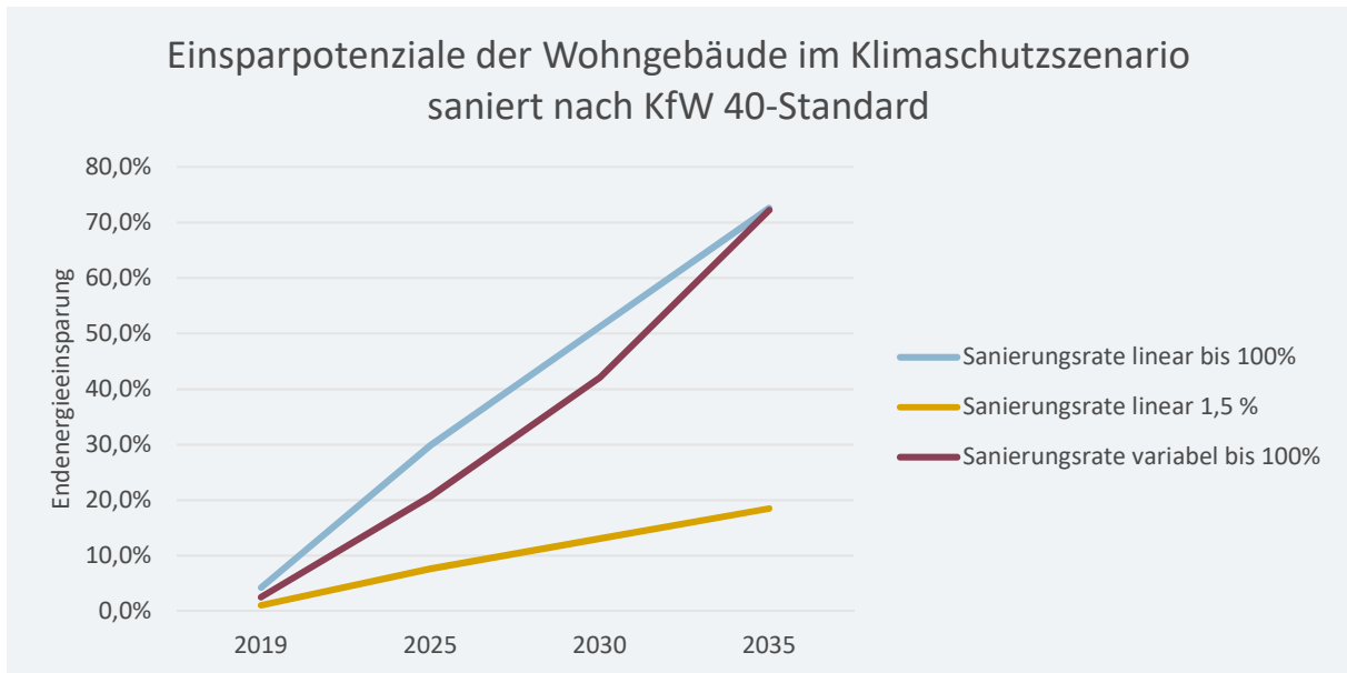
Abbildung 4-74: Einsparpotenziale der Wohngebäude „Klimaschutzscenario2035“ (KfW 40-Standard)“ saniert bis 2035 in der Gemeinde Schwalmtal (Quelle: Eigene Darstellung)
