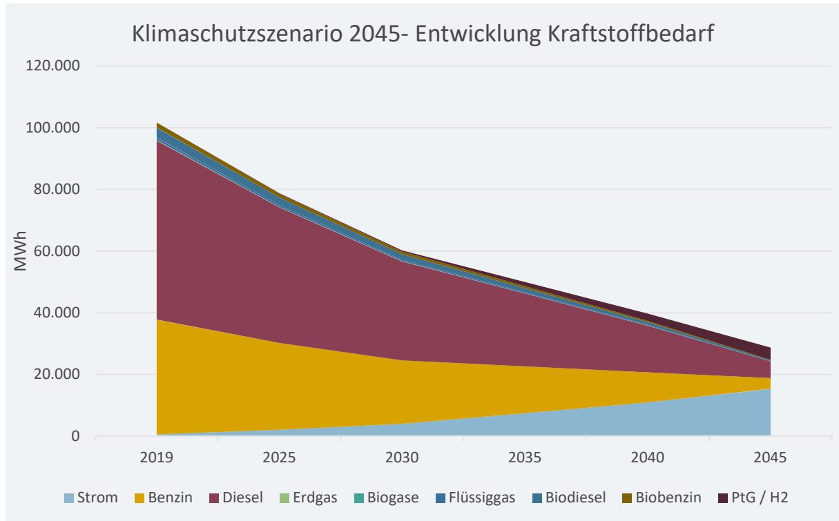
Abbildung 5-70: Zukünftiger Kraftstoffbedarf im Klimaschutzszenario 2045 in Tönisvorst (Quelle: Eigene Darstellung)
